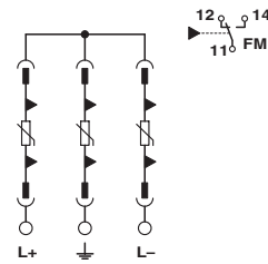
Anschluss des Fernmeldekontakts am Überspannungsschutz
