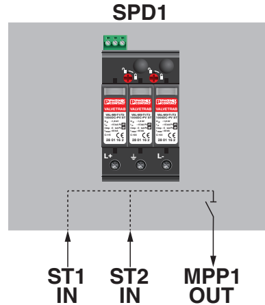
Anschlusszeichnung
