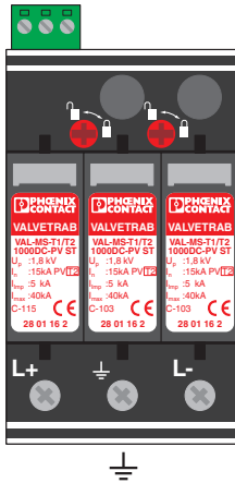
Anschluss des Schutzerdungsleiters am Überspannungsschutz
