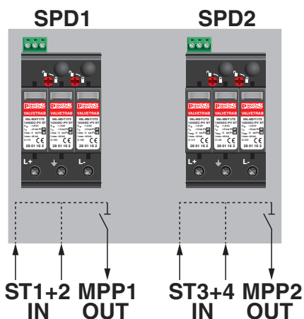
Schematische Applikationszeichnung
