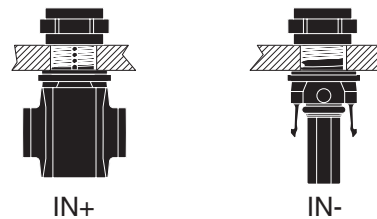
Schemazeichnung
