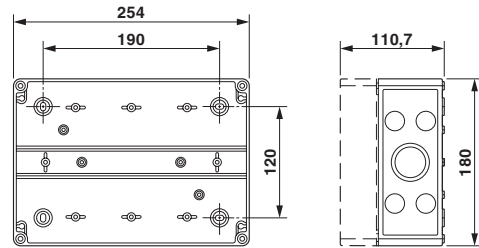
Maßzeichnung
