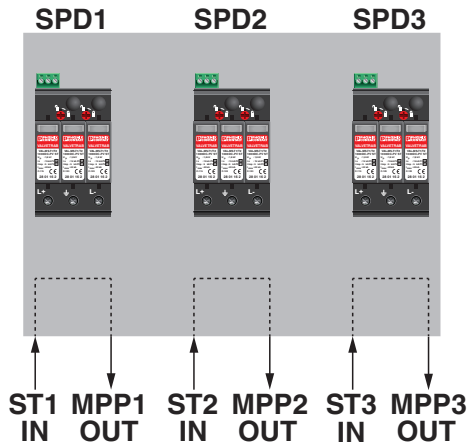
Schematische Applikationszeichnung
